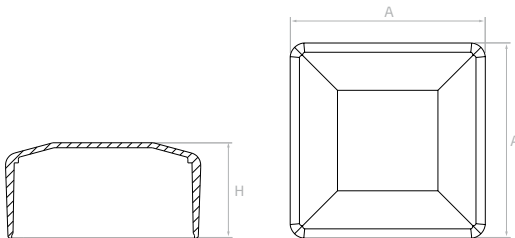
Zaślepka do profilu kwadratowego End cap / Заглушка профиля / Torprofilabdeckung
