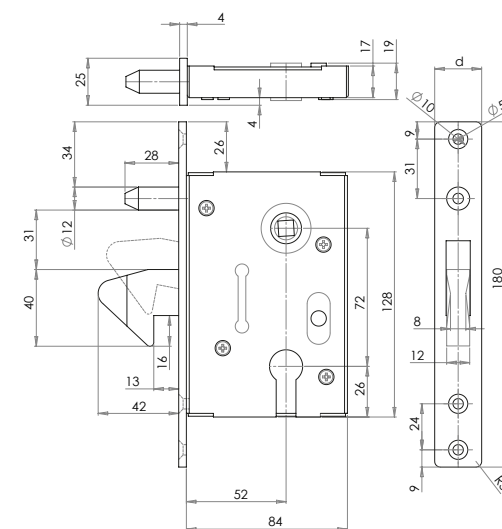
Zamek hakowy Lock / Врезной замок / Hackenschloss
