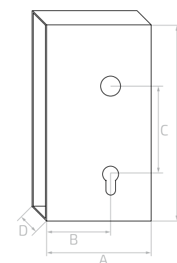
Obudowa zamka Lock box / Корпус замка / Schlosskasten
