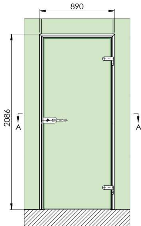
SECTION A-A
